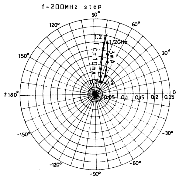
S12e : VCE=10V
