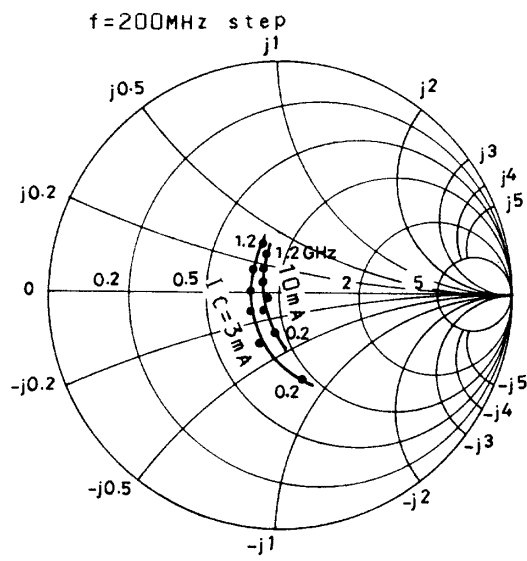
S11e : VCE=10V
